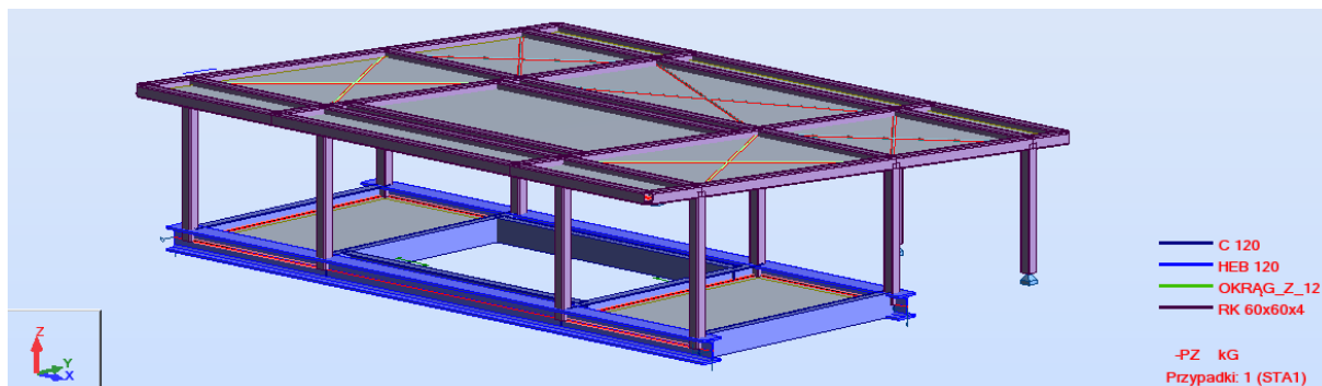
Model obliczeniowy zadaszania stalowego w osiach 4-5/A-B z oznaczeniem profili
