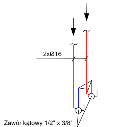
SCHEMAT PODEJŚCIA DO ZAWORÓW CZERPALNYCH
