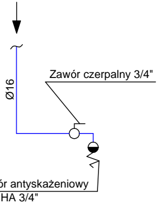
SCHEMAT PODEJŚCIA DO ZAWORÓW CZERPALNYCH
